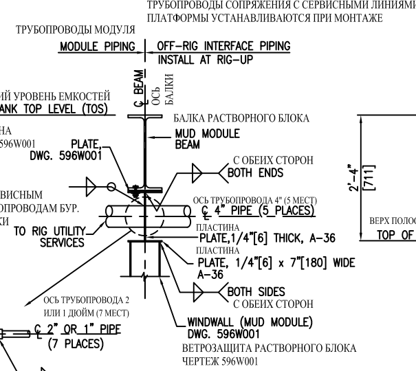
SECTION "2-2" СЕЧЕНИЕ 2-2
