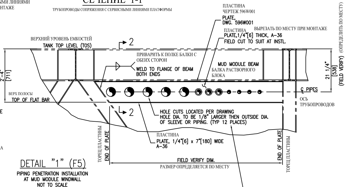
ДЕТАЛЬНЫЙ ВИД 1 (F5) МОНТАЖНЫЕ УЗЛЫ ПРОХОДОВ ДЛЯ ТРУБОПРОВОДОВ В ВЕТРОЗАЩИТЕ РАСТВОРНОГО БЛОКА НЕ В МАСШТАБЕ
